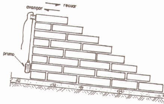
Figura 3 - Detalhe do prumo das alvenarias.
