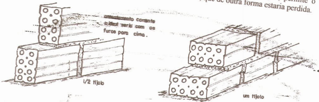
Figura 1 - Execução de alvenaria utilizando tijolos furados.
