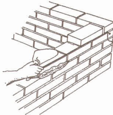
Figura 5 - Assentamento do tijolo
