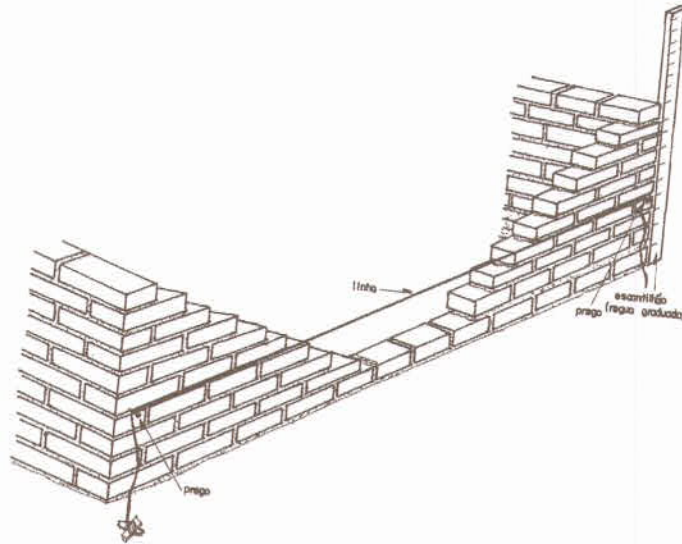
Figura 2 - Detalhe do nivelamento da elevação da parede.
