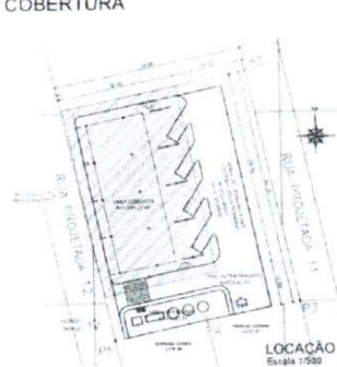
LOCAÇÃO Escala 1/500
