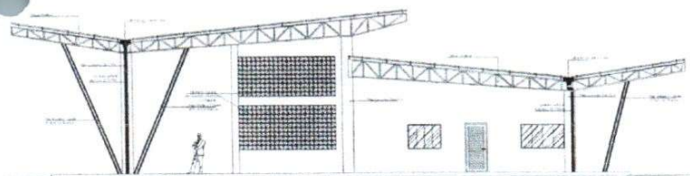
ELEVACÃO D Escala 1:50
