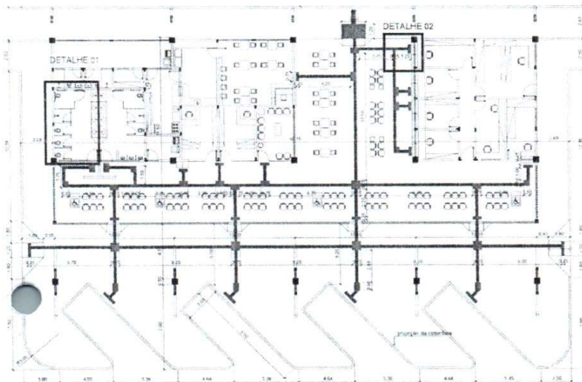
PLANTA DE ACESSIBILIDADE - PISO TÁTIL Escala 1:100
