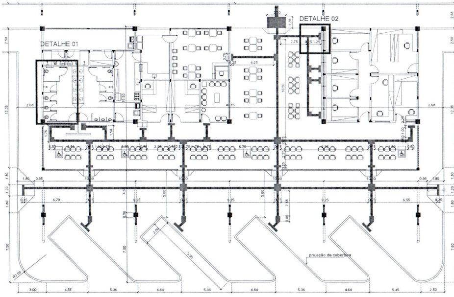
PLANTA DE ACESSIBILIDADE - PISO TÁTIL Escala 1:100
